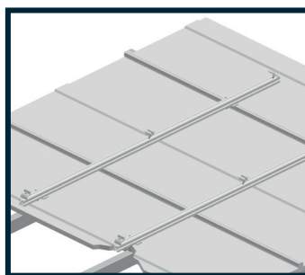
Instalação em cobertura «sandwich»
