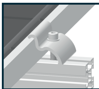
Aperto lateral do painel
