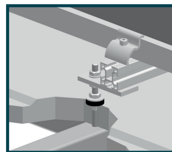
Aplicação do perno de rosca dupla
